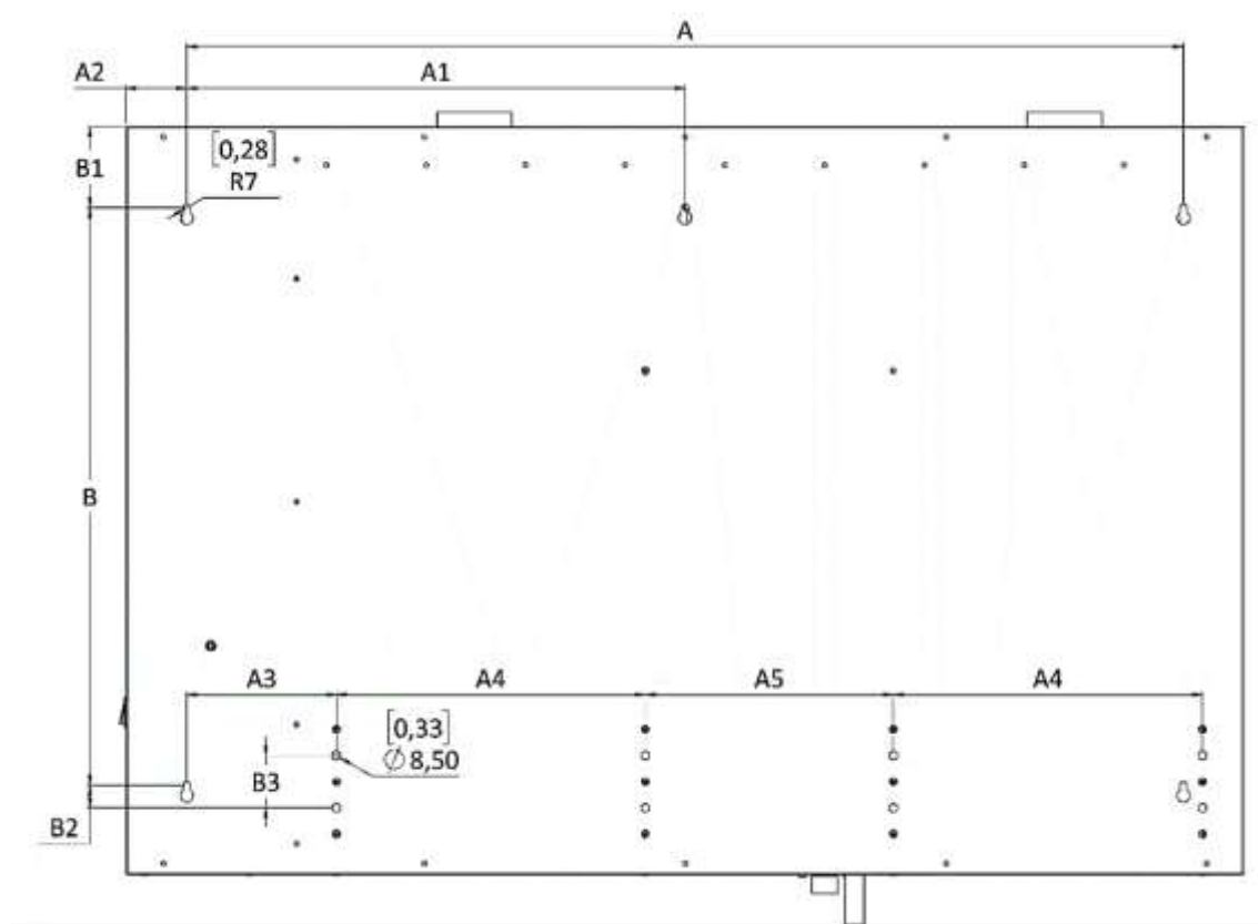
Fig. 3-1. Emplacement trou de fixation
