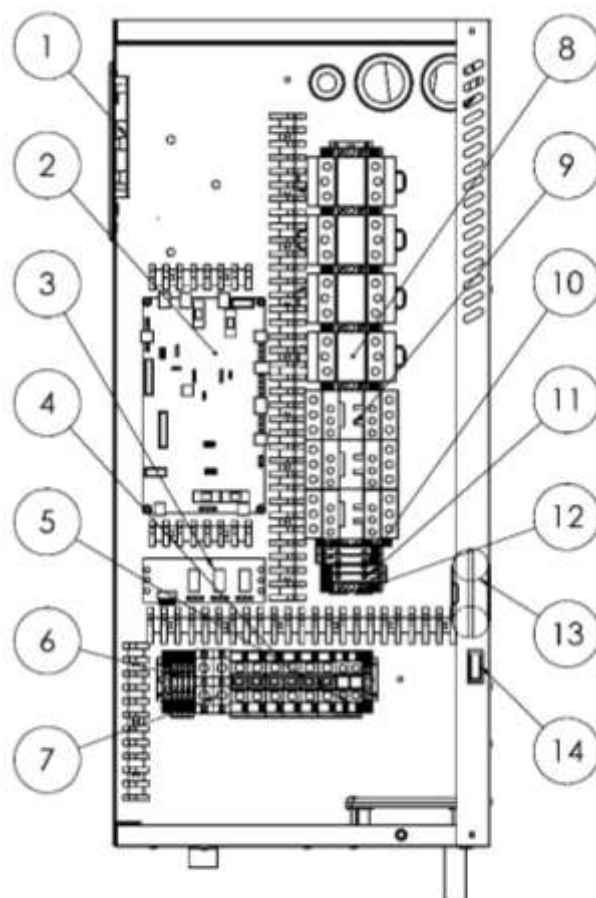
Fig. 7-5. Compartiment électrique
