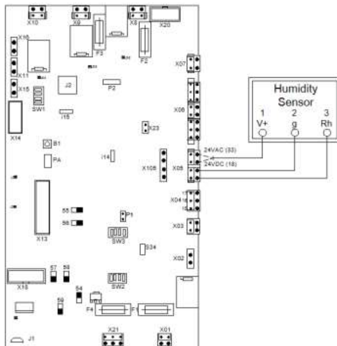
Sonde d'humidité avec alimentation 24VDC (18,19 ,20) ou 24 VAC (33,19,20)
