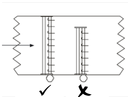
Illustration 3-6. Tout flux d'air doit être redirigé à travers l'ExpressPack®. Si l'ExpressPack® est plus petit que la section transversale du conduit, il devra être positionné au centre du conduit et tous les espaces ouverts devront être obstrués.
