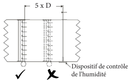
Illustration 3-5. Si vous installez un dispositif de contrôle de l'humidité, veuillez respecter une distance de sécurité de 5 \times D , entre le dispositif et l'ExpressPack®. «D» étant la distance d'absorption.
