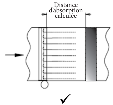
Illustration 3-3. Pensez à respecter la distance définie par calcul entre l'ExpressPack® et le premier obstacle ou transition de gaine.
